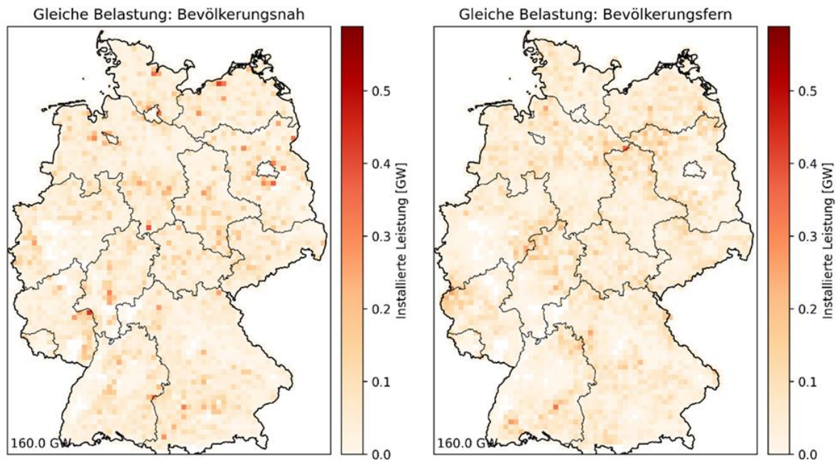
Abbildung 11: Wind Onshore Verteilungen für Deutschland auf Rasterebene – Bevölkerungsnah und Bevölkerungsforn im Vergleich
