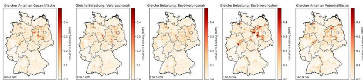
Abbildung 15: Deutschlandweite Ausbauempfehlungen für Wind onshore auf Gemeindeebene je Gerechtigkeitsmetrik
