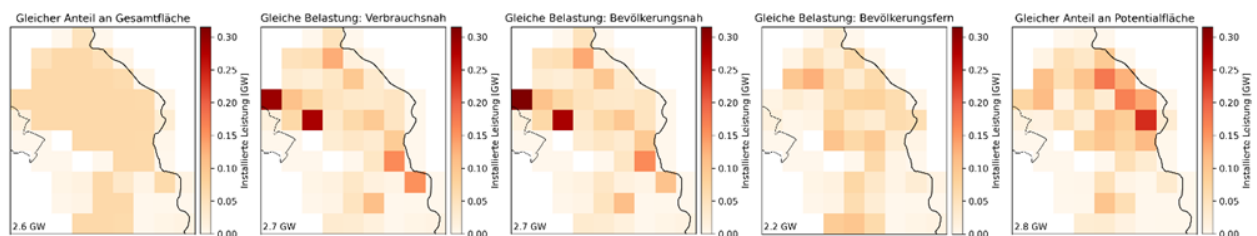
Abbildung 12: Wind Onshore Verteilungen für Oderland-Spree auf Rasterebene
