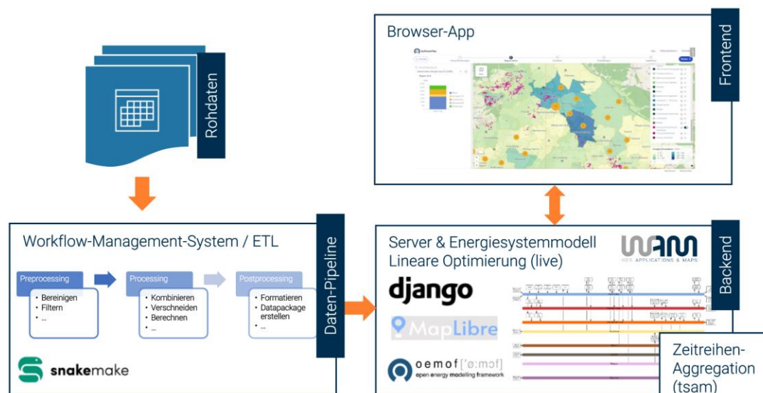
Abbildung 5: Komponenten der Datenaufbereitung und Webapplikation
