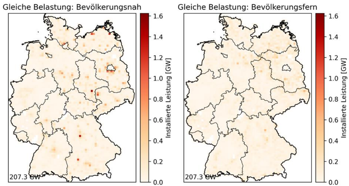
Abbildung 13: PV-FF Verteilungen für Deutschland auf Rasterebene – Bevölkerungsnah und Bevölkerungsfern
