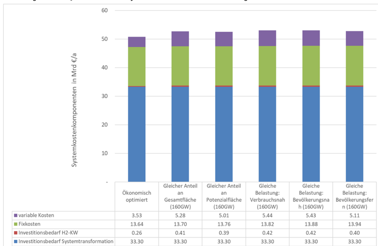
Abbildung 19: Set 1: Jährliche Gesamtsystemkosten der Szenarien im Vergleich
