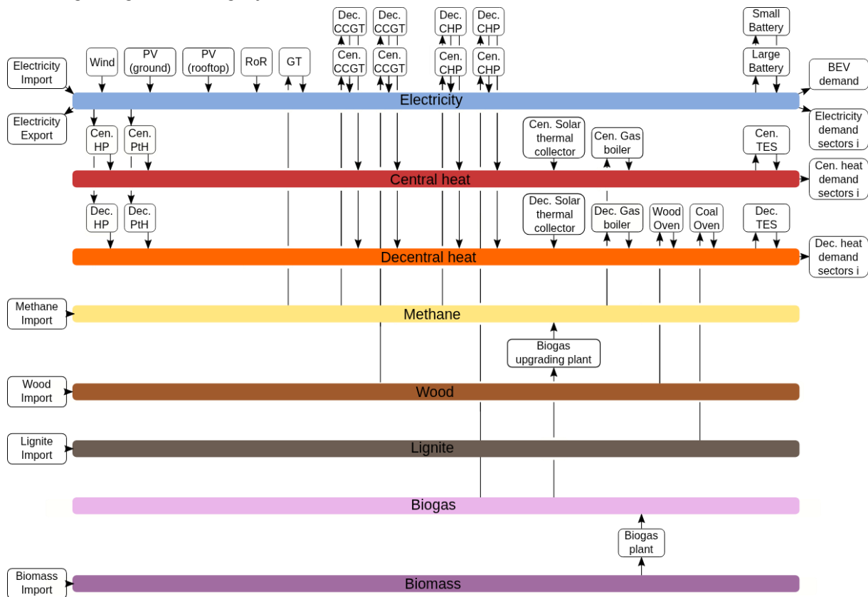
Abbildung 9: Regionales Energiesystemmodell
